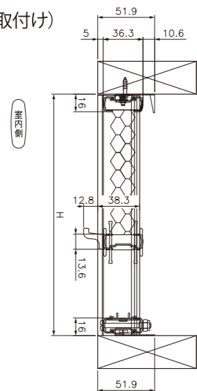
◎横断面図 (窓枠内取付け)
