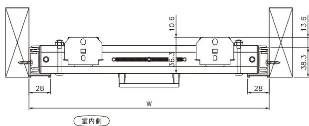
◎横断面図 (窓枠内取付け)
